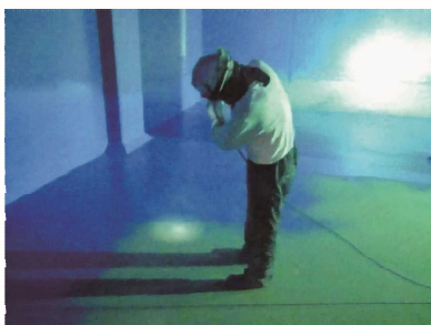
防食材(ナルコート)塗布状況
